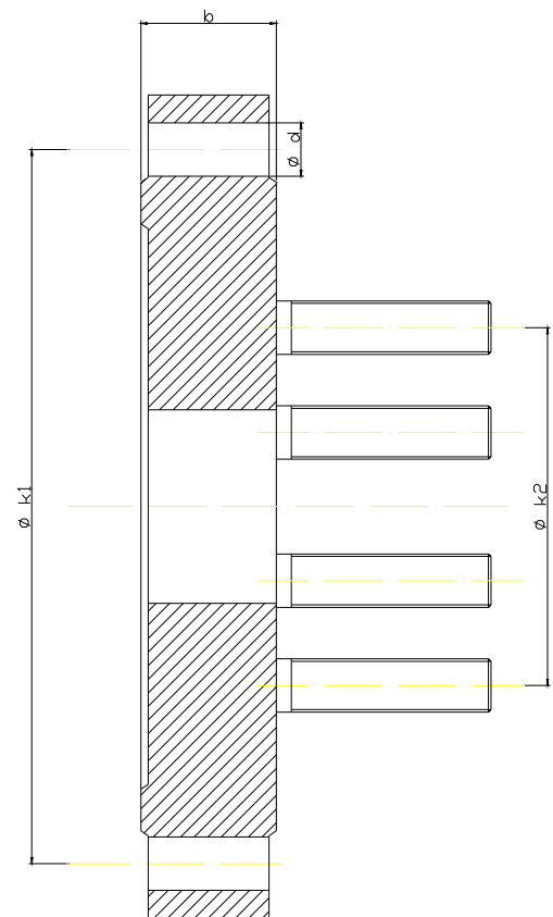
Kołnierze redukcyjne typ B
