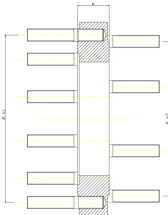
Kołnierze redukcyjne typ A
